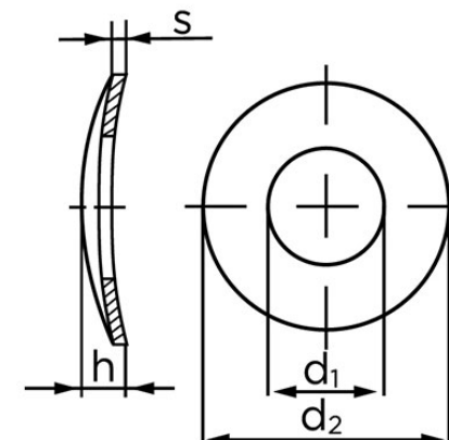
DIN 137 B
