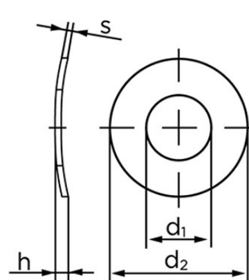
DIN 137 A
