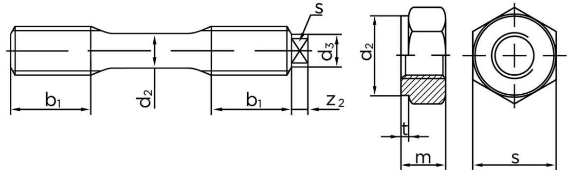
DIN 2510 L
