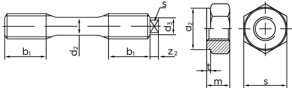
DIN 2510 L
